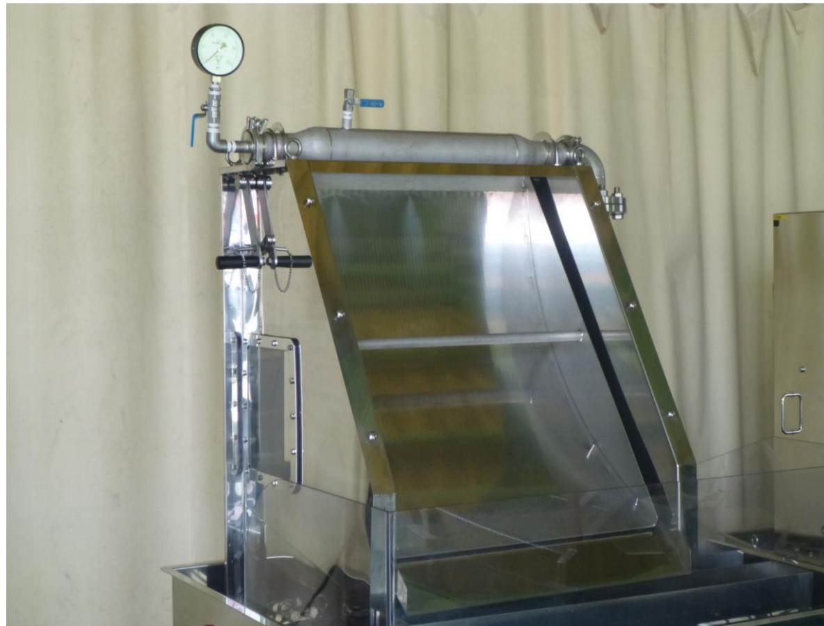
30 \mu mスリットのファインウェッジを用いた固液分離装置 「ファインアルジ」
